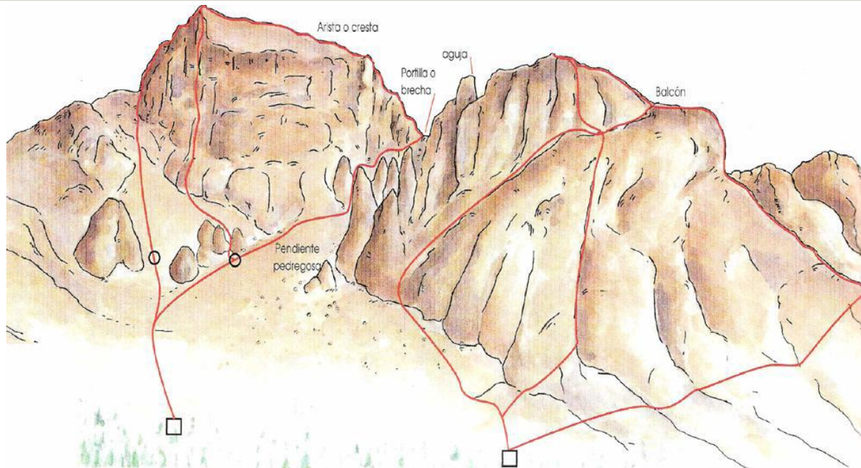
Esquema que muestra algunas características principales de una montaña.
