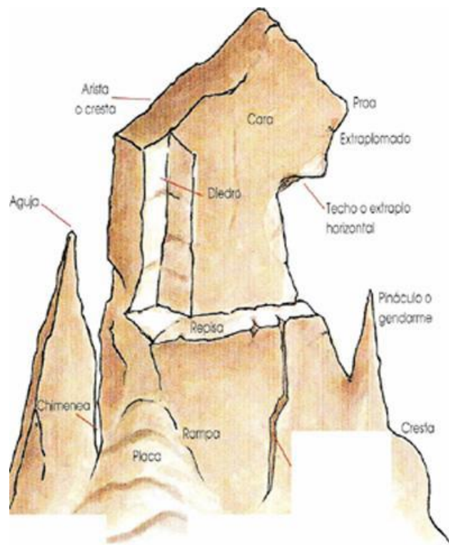
Características de un Peñasco Rocosó.
